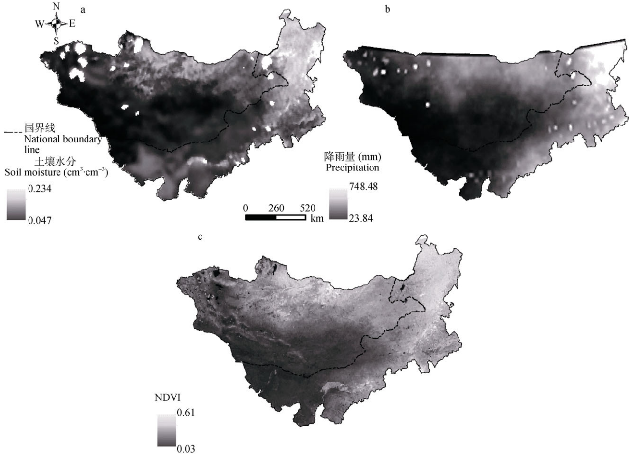
图 3 蒙古高原植被生长期土壤水分、降雨量及平均植被指数空间分布
